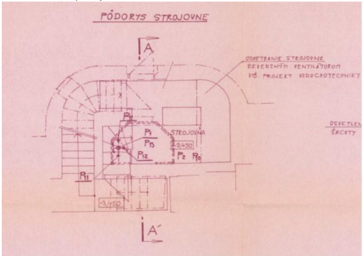
Obrázok č.5: Pôdorys strojovne
