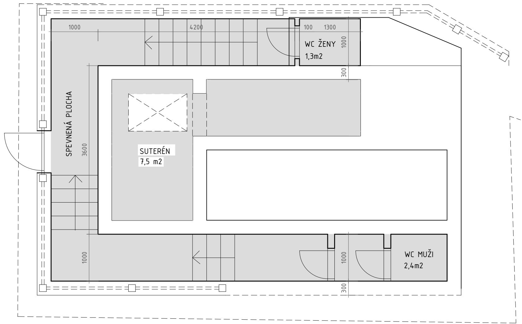
Pôdorys 1.PP
