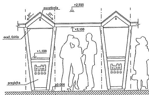
ČELNÝ POHĽAD (rozvinutý)
