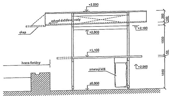
REZ A-A (výřez)
