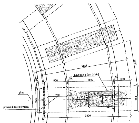
PÓDORYS (výřez)
